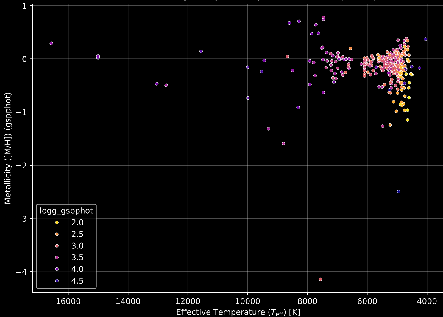
APOGEE DR17 Field: [266-06] Stellar Population Parameters (n= 373)
